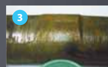
Дефектный неоригинальный вал
