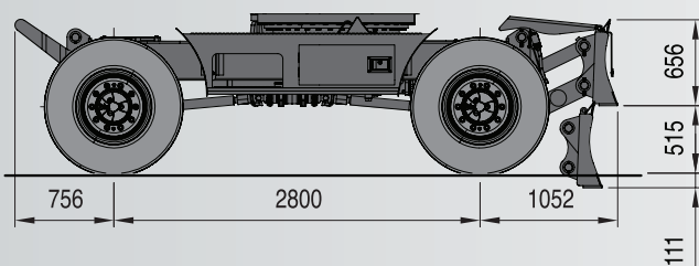
▲ Переднее гнездо транспортного крепления стрелы и задний отвал
