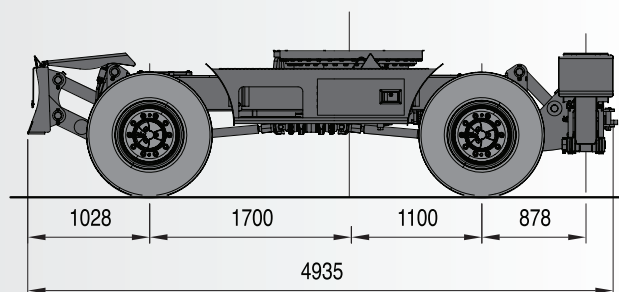
▲ Передний отвал и задний отвал
